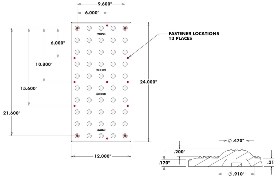
SECTION A-A
