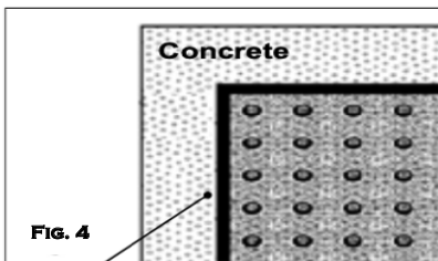
FIG. 4 1/8" Deep Troweled Edge
